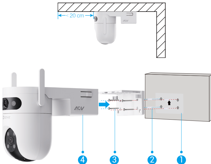
Figura 2. Montaje en pared
